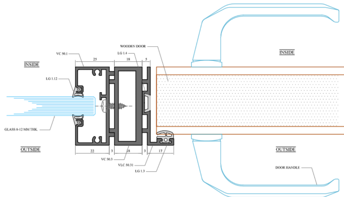
VICO DOOR PLAN
